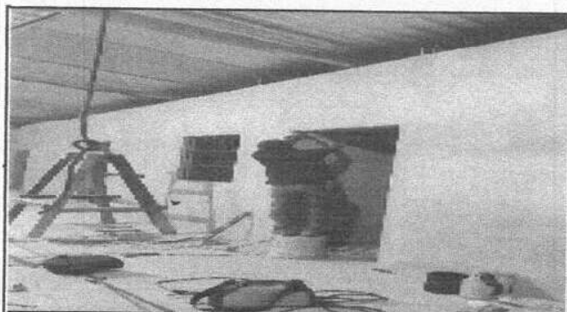
Foto 3: MODULO 1. STITUCION DE PUERTA DE MADERA POR METAL CON CHAPA E INSTALACION DE VENTANA DE METAL CON VIDRIO.
