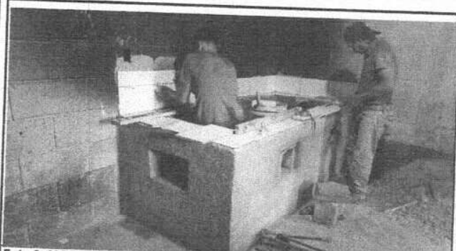
Foto 3: MODULO 3. CONSTRUCCION DE ESTUFA RURAL E INSTALACION DE AZULEJO.
